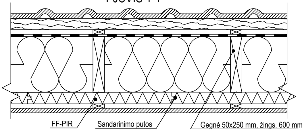
PJŪVIS 1-1
